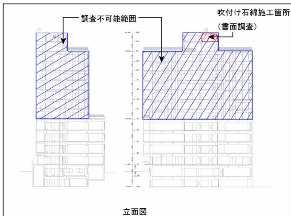
資料 C 建築物の構造と見取り図(調査不可能場所と石綿施工箇所)(例)
